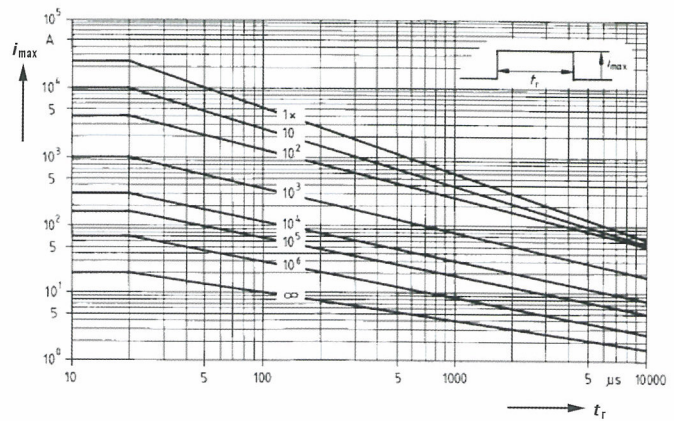
MYE30-201□ ~ MYL30-122□
