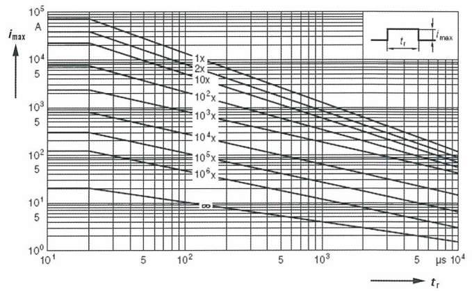
MYE70-201□ ~ MYL70-472□
